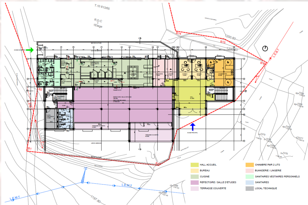
Plan RDC
