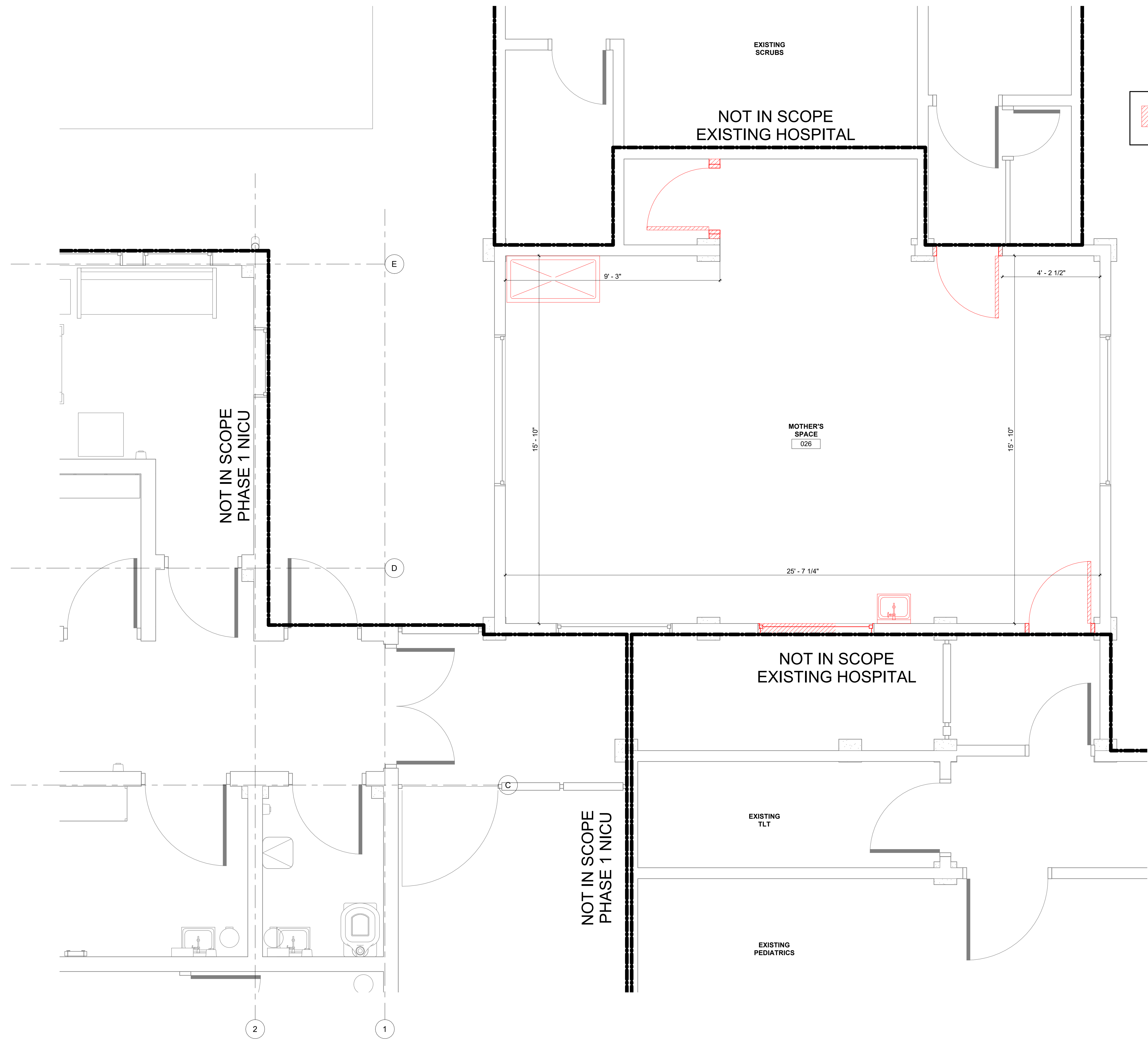
1 PHASE 2 DEMO PLAN SCALE 1 : 25
