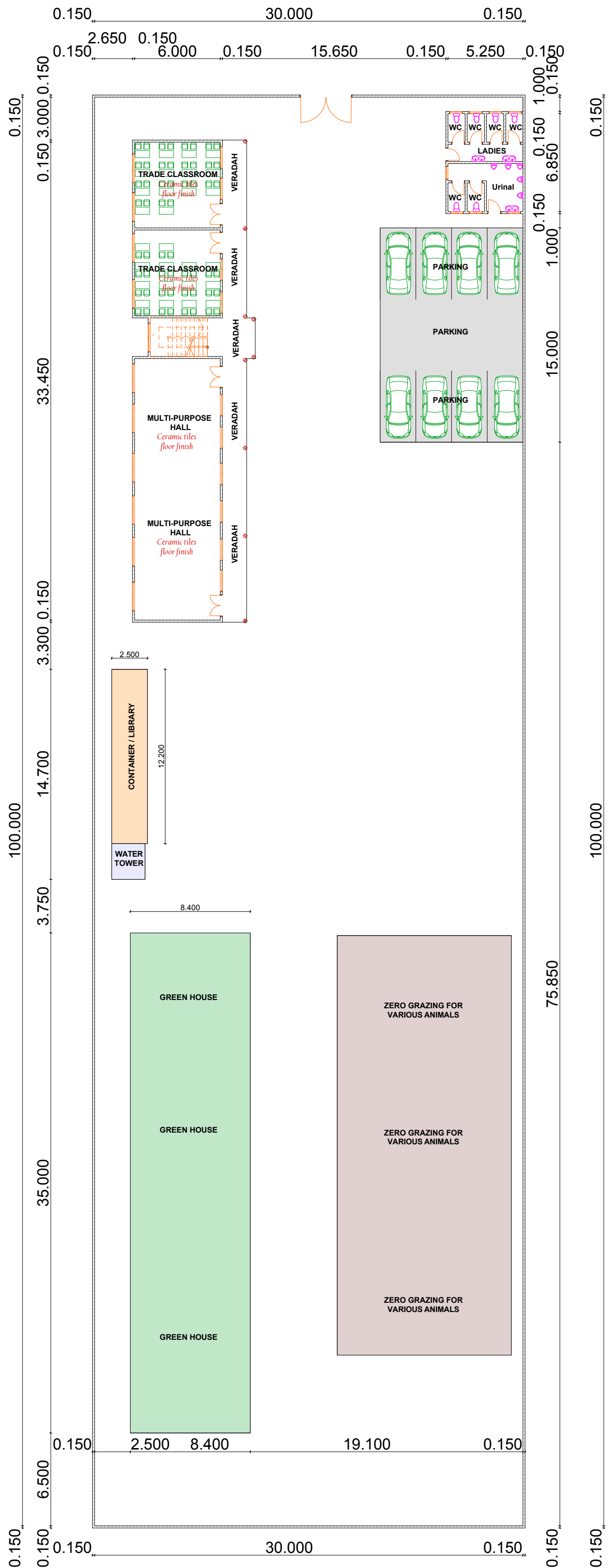
SITE PLAN LAYOUT.
