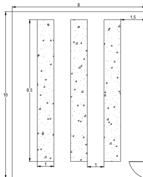
Vista en Planta camas de germinación
