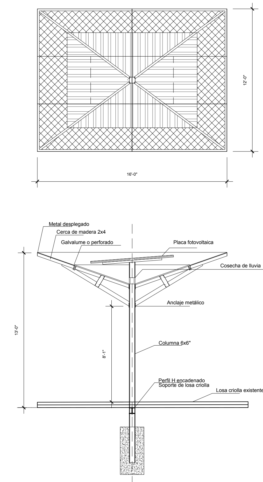
DETALLE COLUMNA
