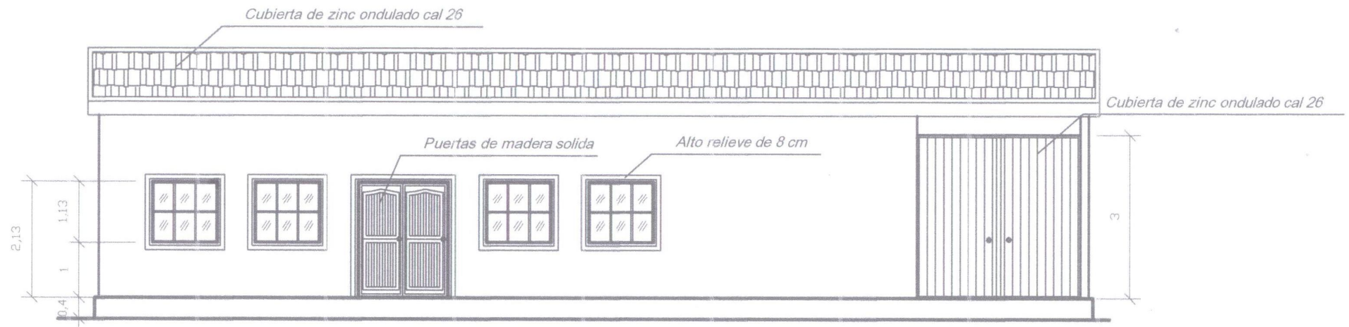
ELEVACION PRINCIPAL
